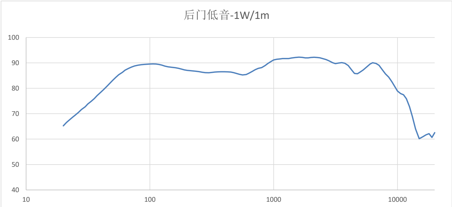
频响曲线
