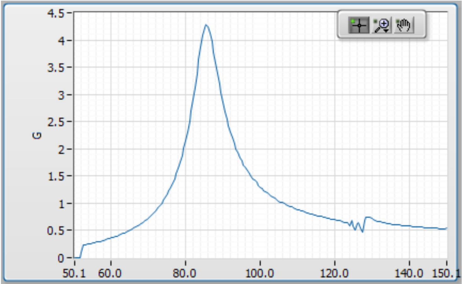
频响曲线
