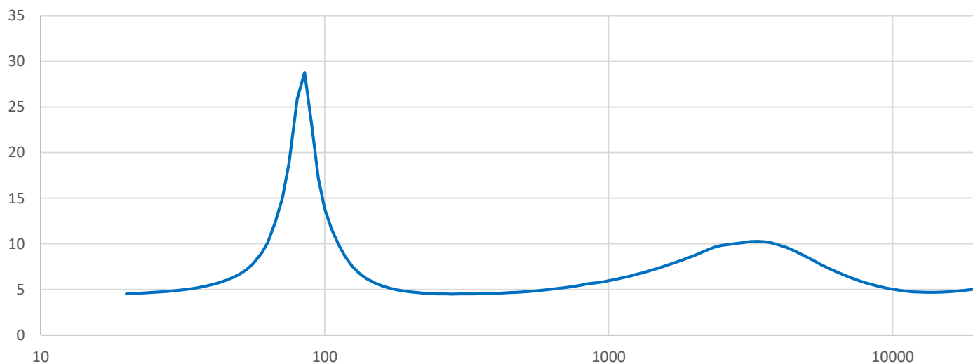
同轴扬声器-1W/1m
