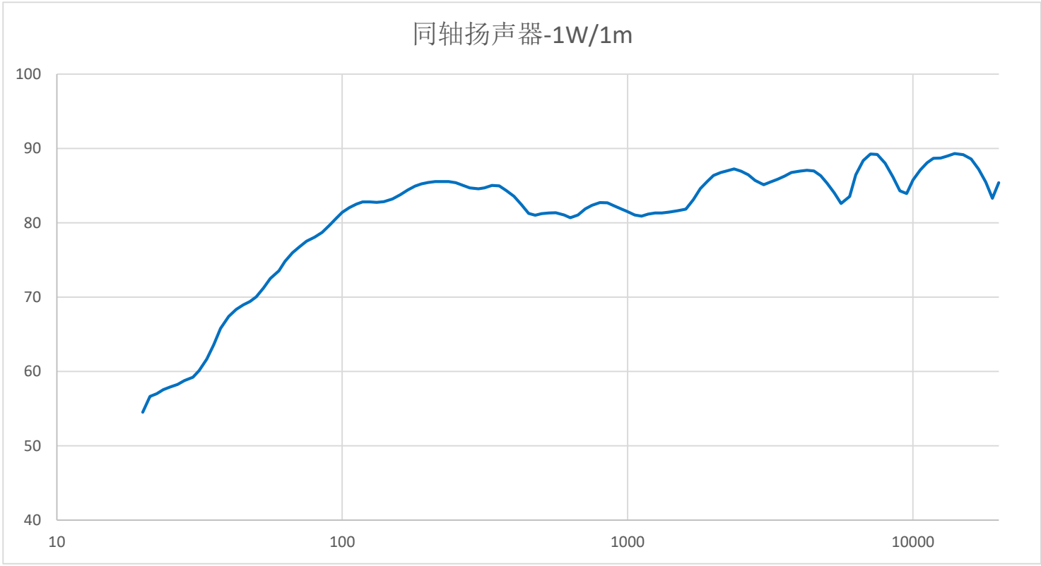
频响曲线
