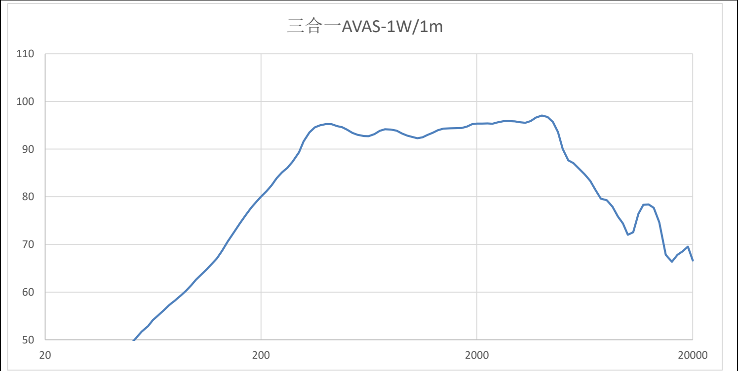
频响曲线
