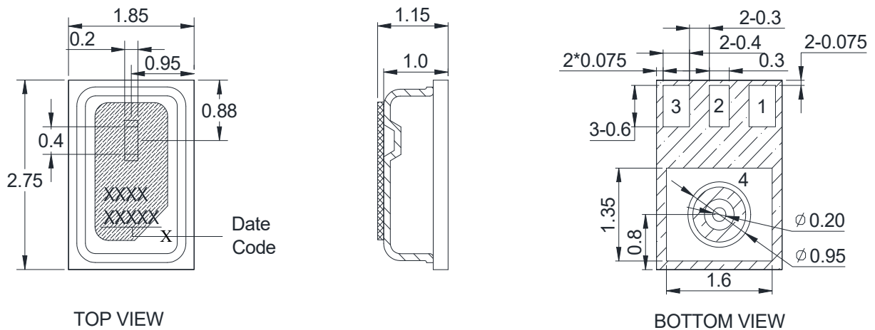
图 2 尺寸图
