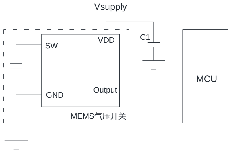
图 3 应用电路
