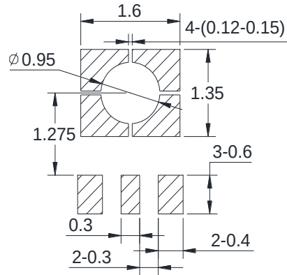
图 8 推荐锡膏印刷板设计
