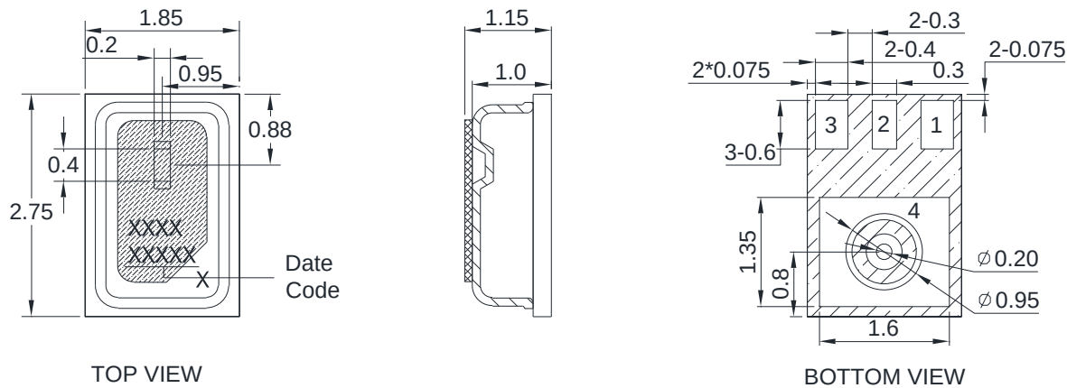
图 2 尺寸图
