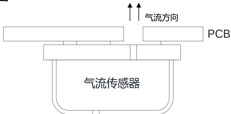
图 4 组装示意图
